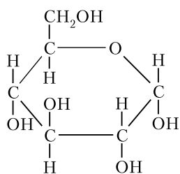
Глюкоза
