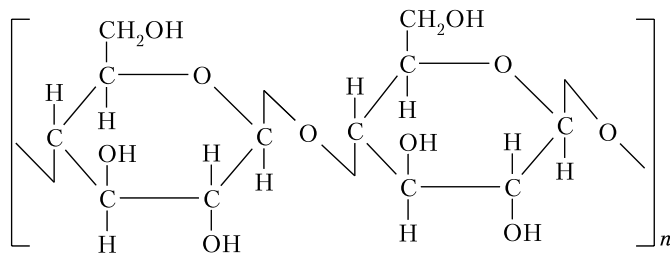
Целлюлоза
