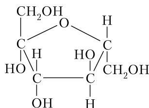
Фруктоза
