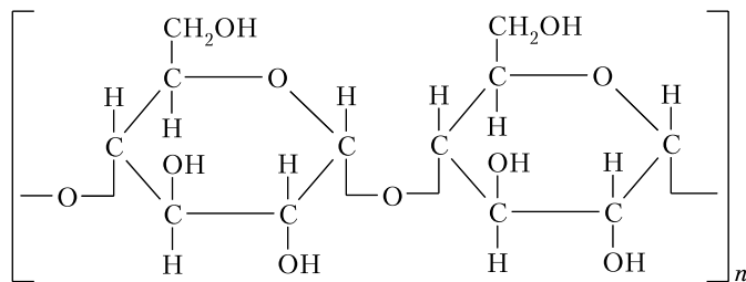
Крахмал
