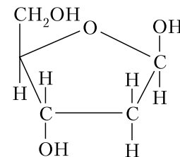
Дезоксирибоза
