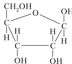
Рибоза
